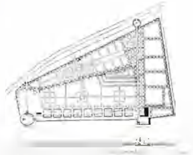
Fig. 35. Nya begravningsplatsen i Simrishamn. Arkitekt Markelius. Anläggningen under utförande. Medelst trädramar bildas tvenne långsträckta gårdar, som återigen uppdelas av tuktade häckar i mindre gravfält. I bildens högra sida trädramas mindre gravgårdar. Längst till vänster på bilden synes läget för ceremoniplatsen inom mycket högväxande tuktade häckar. Mindre traditionsbunden komposition jämfört med Malmöanläggningen.
