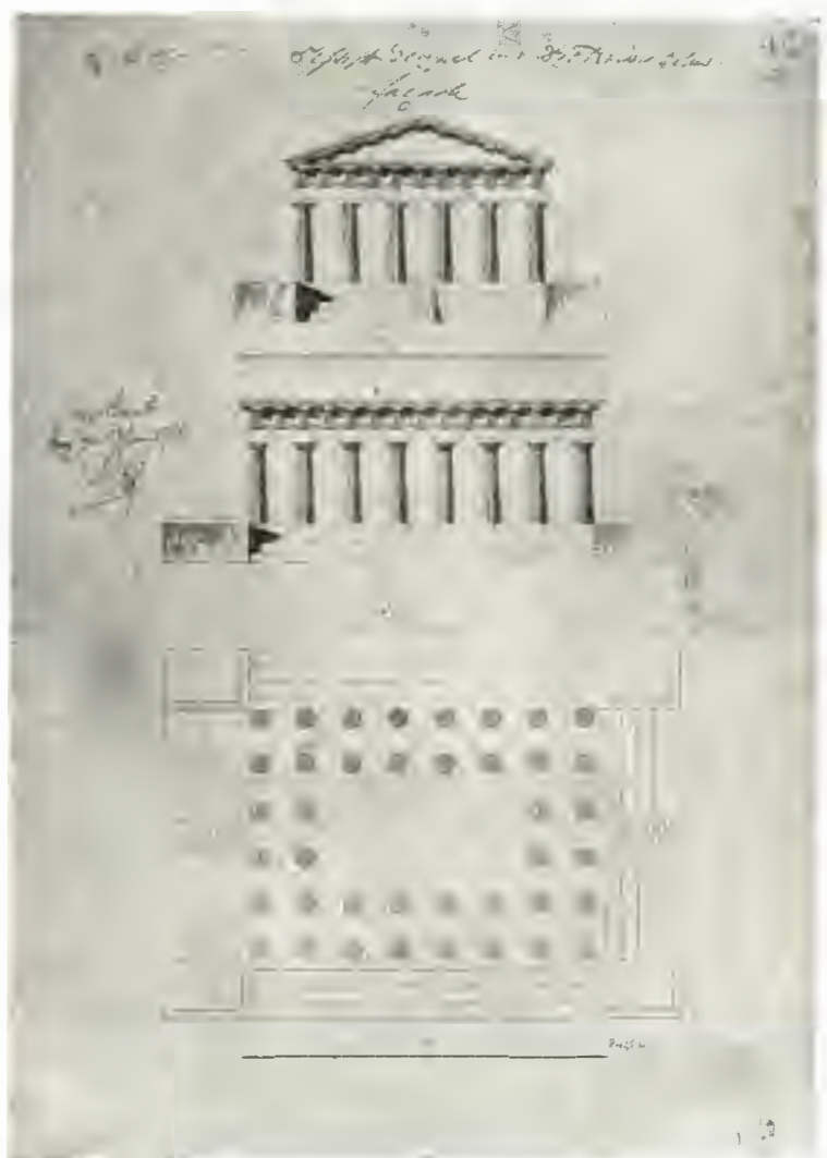
Fig. 85. Drottningholm. Prästiskt tempel. Projekt av Louis Jean Desprez 1788. Slottsarkivet.
