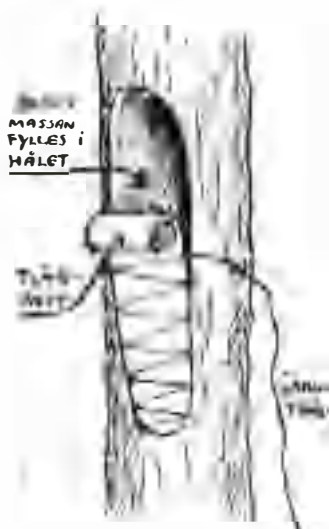
Fig. 2. Medelst tjärpapp göres en vägg, vilken hindrar betongmassan att rinna ut, när stora hål skola plomberas.
