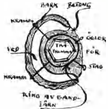
Fig. 8. För att minska betongpelarens tyngd ingjutes en trätrumma. I en järnring fästas öglor, i vilka stagen anbringas.
