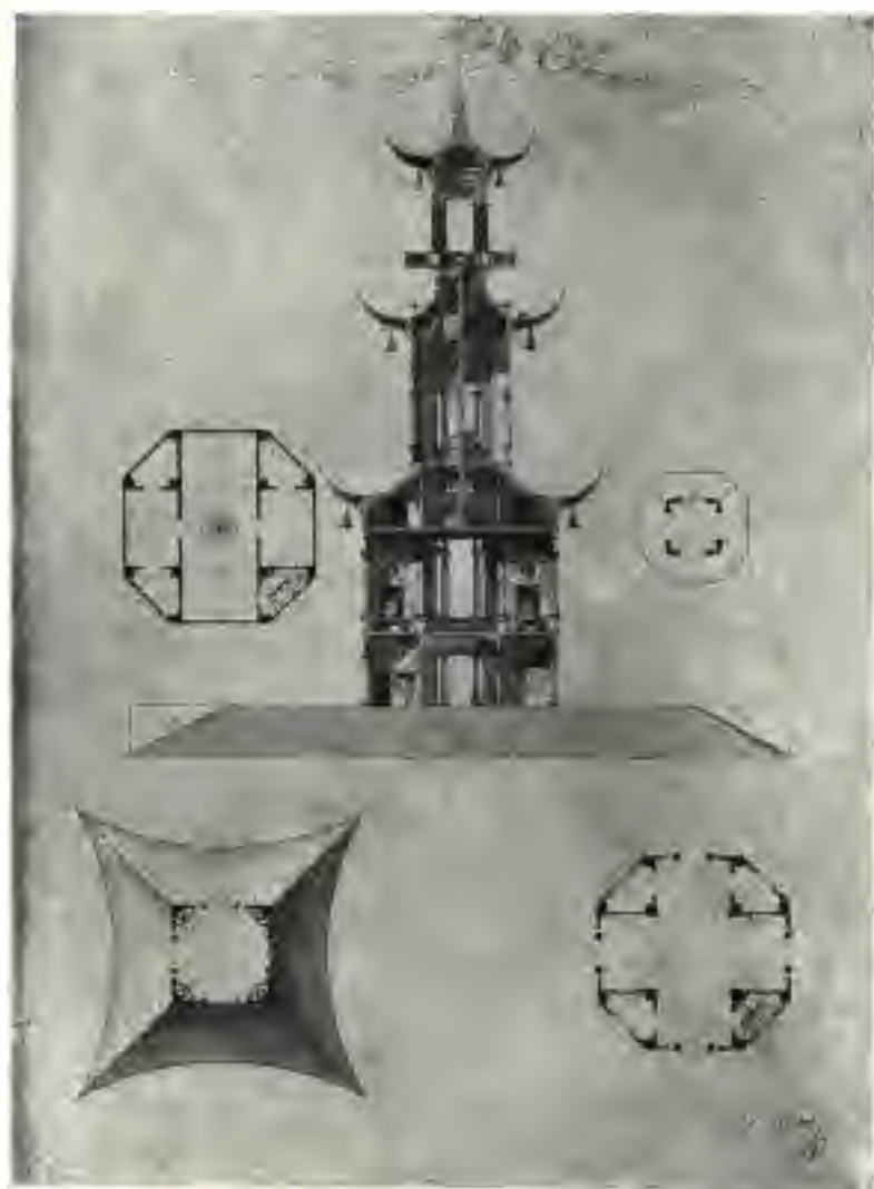
Fig. 83. Drottningholm. Kinesiskt torn. Projekt av Louis Jean Desprez 1788. Slottsarkivet.
